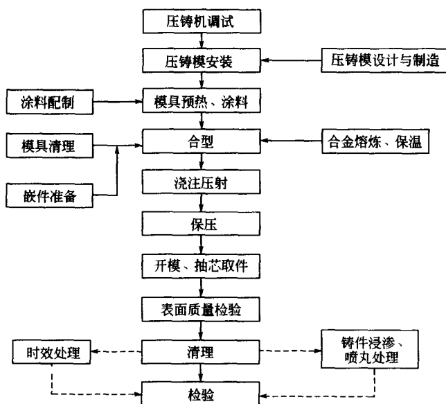
图 1-1 压铸件生产的主要工艺程序
