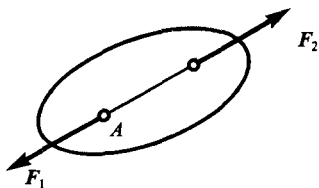
图 1-1 二力平衡
