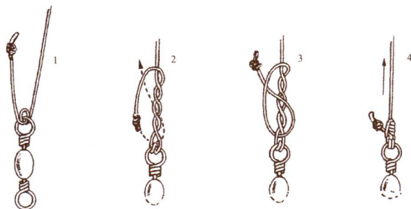
主线与 8 字转环连接
