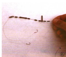
绑上长脑线双钩
