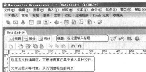
文档编辑区
