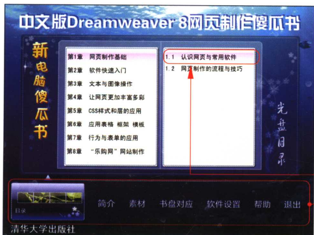
图1 光盘主界面
