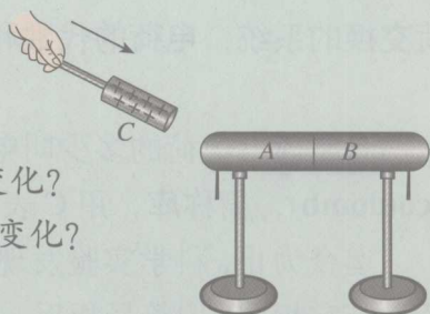
图 1.1-1 静电感应
