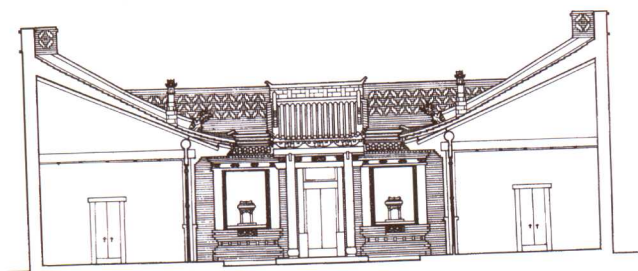
图 611-6 一进院横剖面 宋昆《平遥古城与民居》
