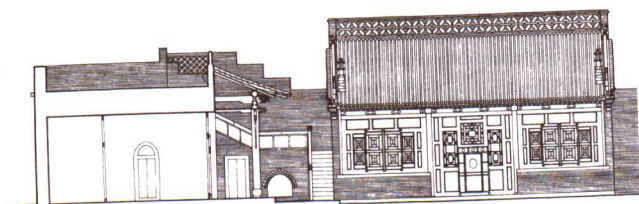
图 611-8 纵剖面 a 宋昆《平遥古城与民居》
