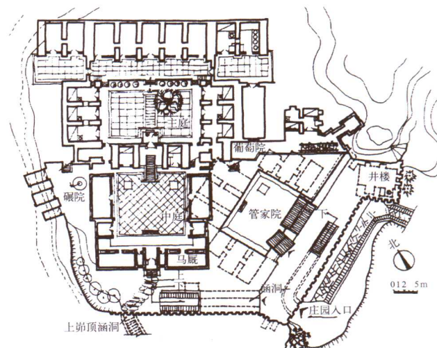
图 611-17 米脂县刘家峁姜园总平面 侯幼彬《中国古代建筑历史图说》
