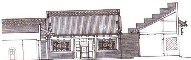
图 611-9 纵剖面 b 宋昆《平遥古城与民居》
