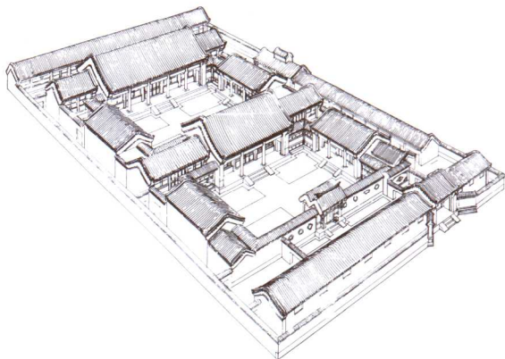
图 611-3 一主一次并列式院落示意图 马炳坚《北京四合院建筑》
