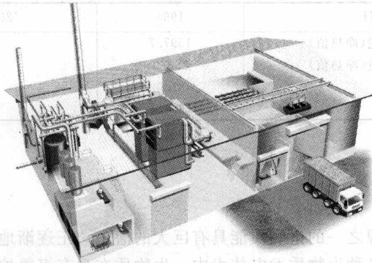
图 1-3 位于瑞典 Wilderswil 的燃木材区域供热厂布局 (感谢 SchmidAG 惠允, 瑞典)
