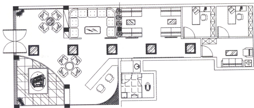
平面布置图
