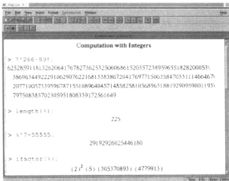
图 1.6.1 Maple 中的整数运算
