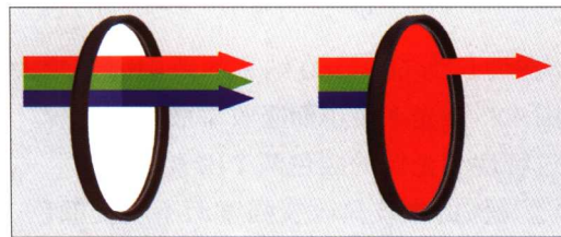
图1-6 透光体对不同波长的光波吸收比例相等时，透过透光体的光波颜色不变（左）；吸收比例不同时，透过透光体的光波改变颜色（右）。
