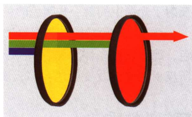
图1-11 颜色的减色效应。
