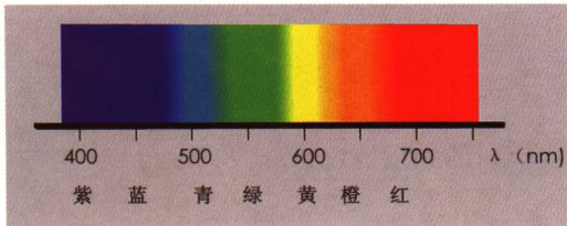
图1-4 可见光的光谱分布。
