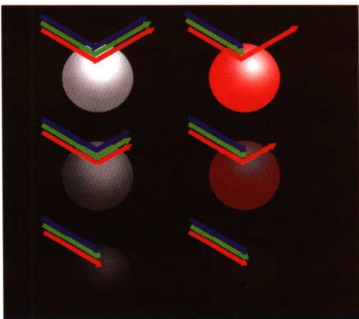
图1-7 反光体对不同波长的光波反射比例相同时,反射光的光波颜色不变(左);反射比例不同时,反射光的光波改变颜色(右)。
