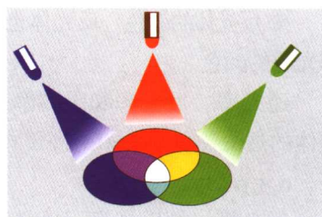
图1-10 颜色的加色效应。
