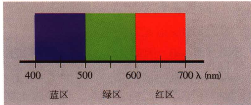
图1-5 将可见光简化为蓝、绿、红3个区域。
