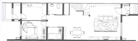
二层平面图
