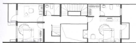
一层平面图
