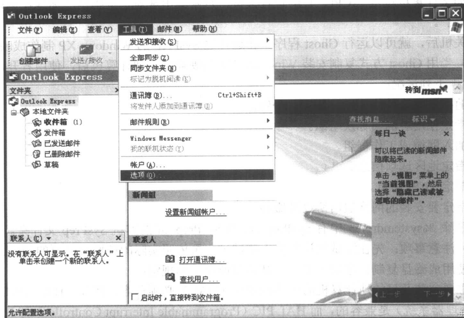
图 1-1 OE 主窗口
