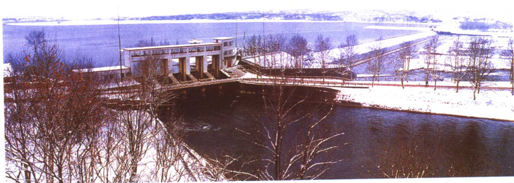
淝河渠首横排头枢纽
