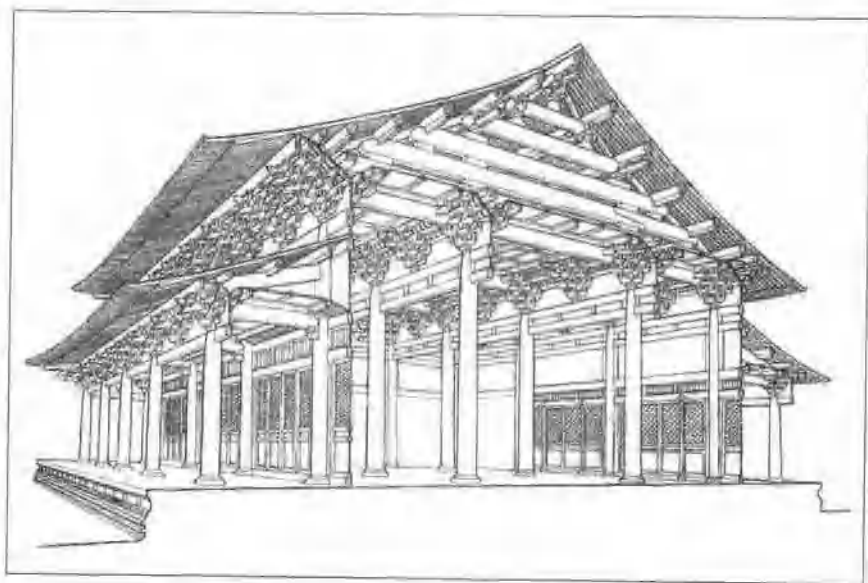
图 0-3 《营造法式》大木作殿堂结构示意图
