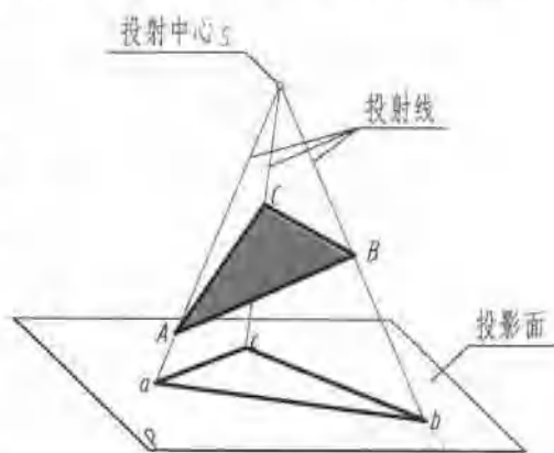
图 1-2 中心投影法
