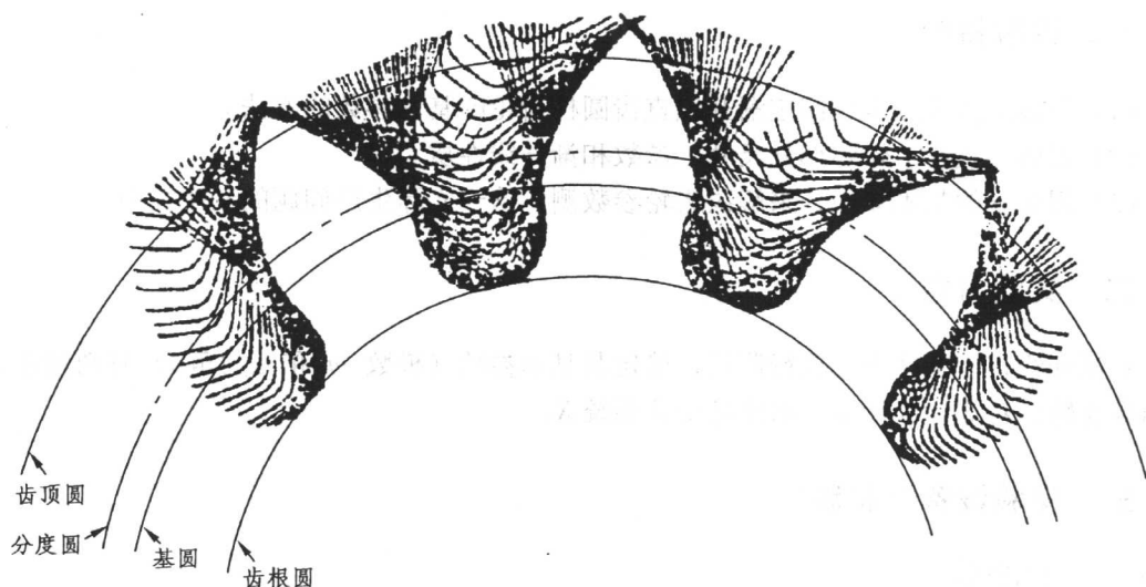
图 2.3 标准齿轮 ( Z=10 )
