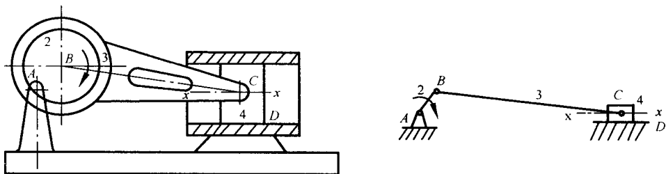
图 1.5 偏心轮机构
