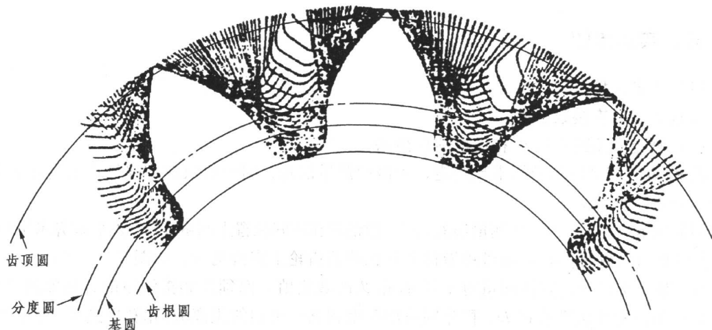
图 2.4 正变位齿轮 ( Z=10, x=0.4117 )
