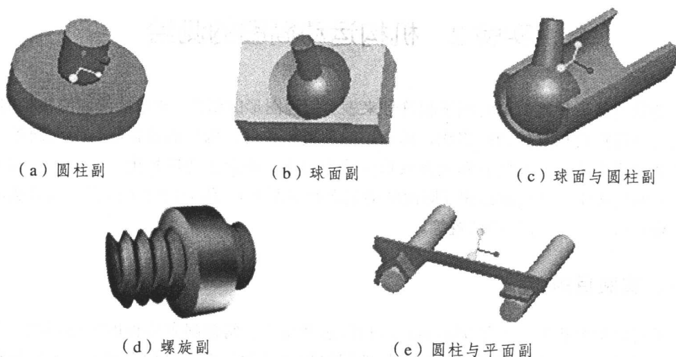
图 1.4 运动副的分类 3
