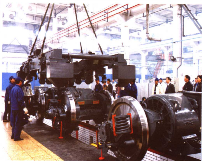
同车转向架作业法
