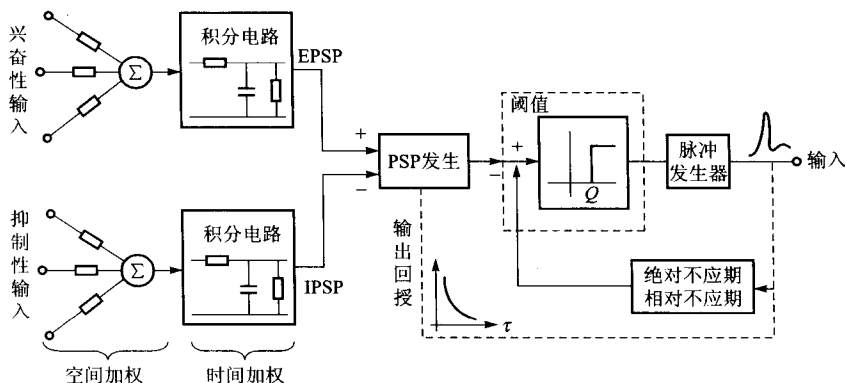
图 1-8 脉冲输出神经元模型功能框图
