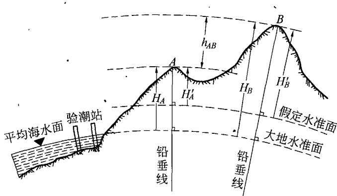
图 1-7 高程与高差的定义及其相互关系
