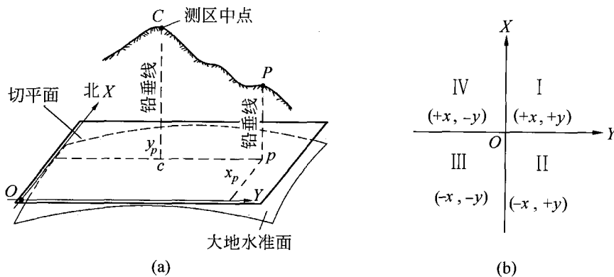
图1-6 独立平面直角坐标系原理图
