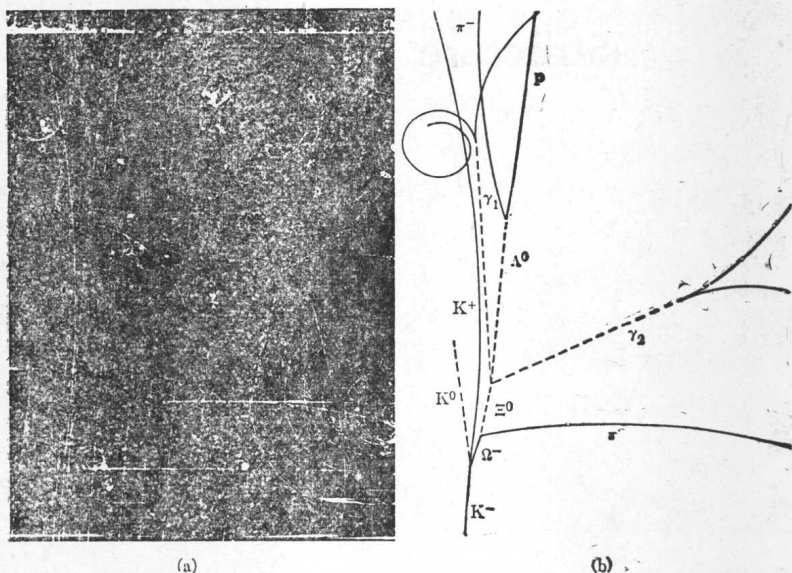
圖 1-1 (a) 在 80 英寸 (2 米) 的液態氫氣泡室內的基本粒子的路線，氣泡室被放在強磁場中，以便驅使帶電荷的質點循曲線路徑而行。先分析這些路線，再由這項分析推出不同粒子的性質。這張 1964 年拍的相片已成歷史。它提供出 \Omega^- 粒子 (英文名字是 omega minus) 存在的第一證據，這種粒子先前已由理論根據預言它的存在。(b) 圖中的線指出相片中所記錄下來的較重要的事件。 \Omega^- 的路線是靠近相片底下的短線，相當於其他各路線的各種質點也都分別得以驗明而標明在圖上。(相片取材自 Brookhaven 國家實驗室)。
