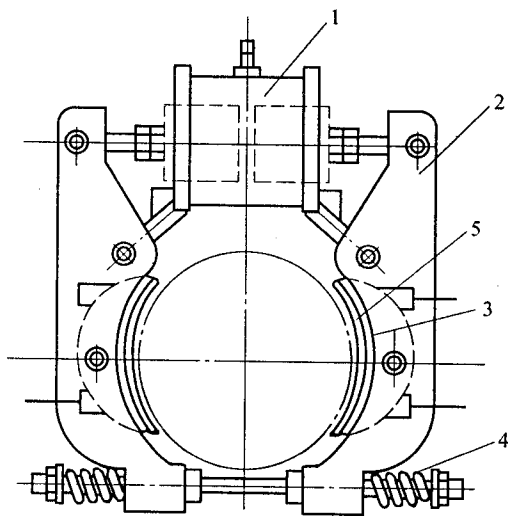
图 1.7 电磁制动器
