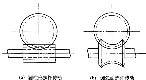
图1.4 蜗杆传动的种类
