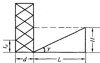
图1.3 蜗杆螺旋升角 \gamma —螺旋升角; t_d —齿距; d —分度圆直径; L —分度圆周长; H —导程
