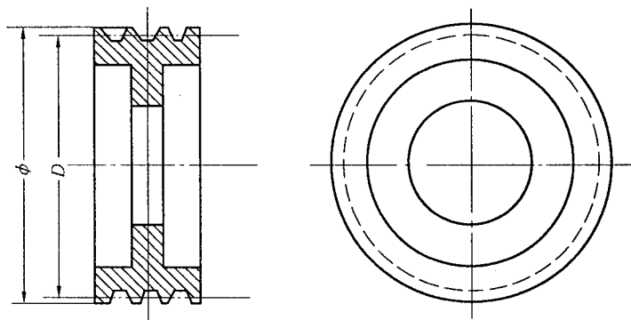
图 1.5 曳引轮
