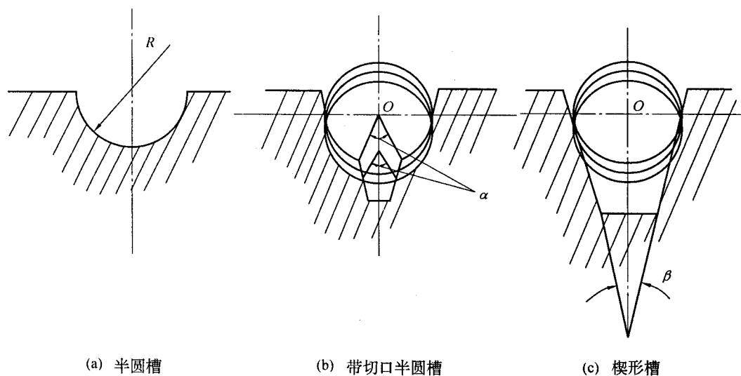
图 1.6 绳槽形状
