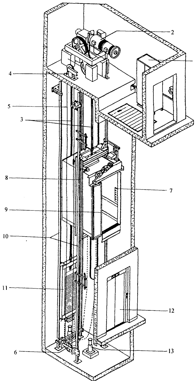
图 1.1 电梯的基本结构
