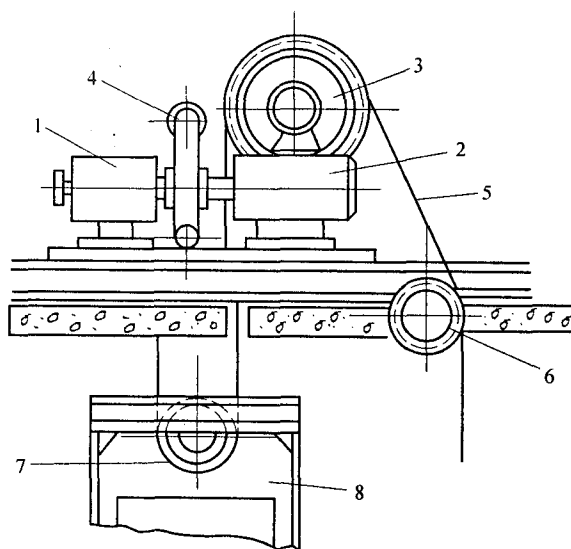
图 1.2 曳引系统
