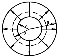
图 1-6 同心圆球电极间电场(内、外球半径分别为 r 、 R )
