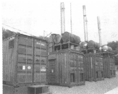
镇江市丹阳镇农村为农户提供燃气的秸秆气化站
