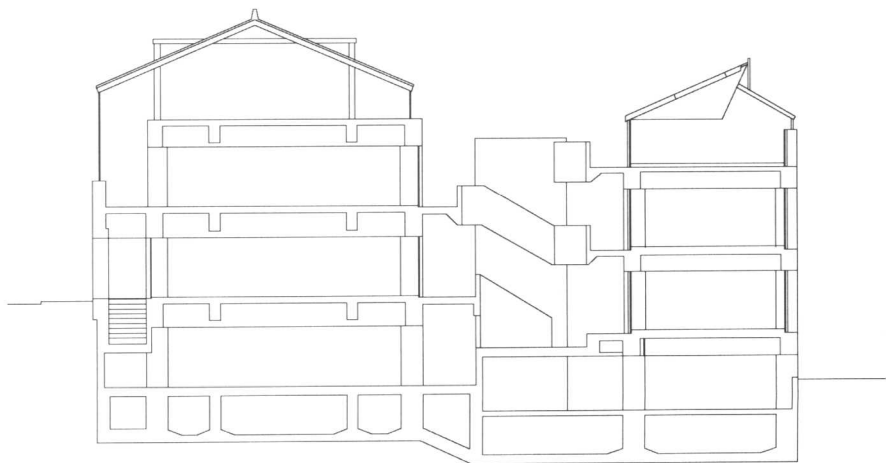
图1-7 从ROSE GARDEN的剖面图可以看到内部的庭院
