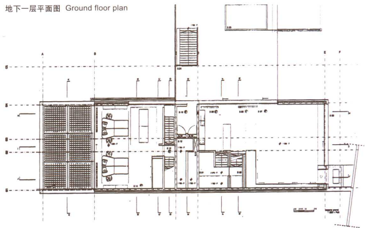
地下一层平面图 Ground floor plan
