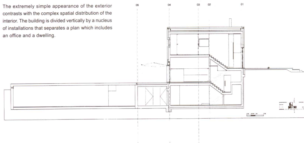
F-F 剖面图 Section F-F
