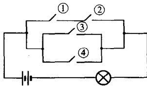
图 1-8 开关电路图
