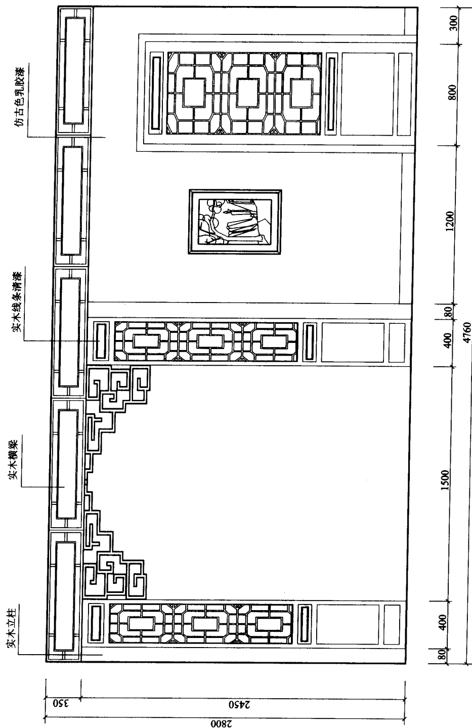
客厅A立面图
