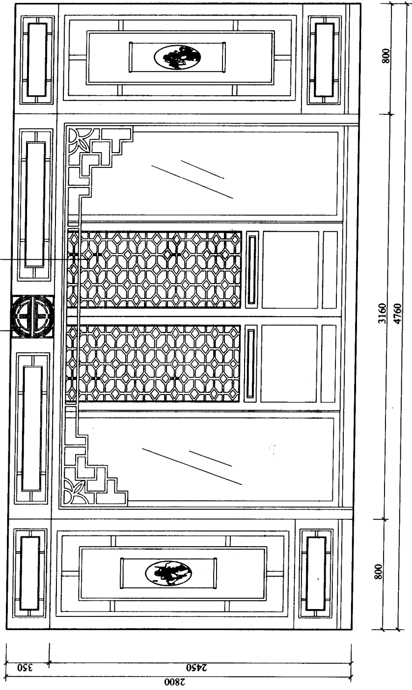
客厅C立面图
