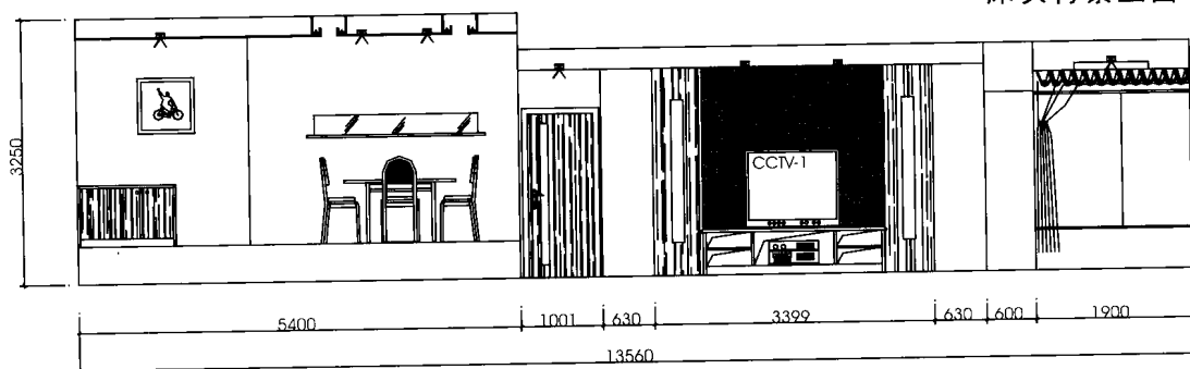
电视墙立面
