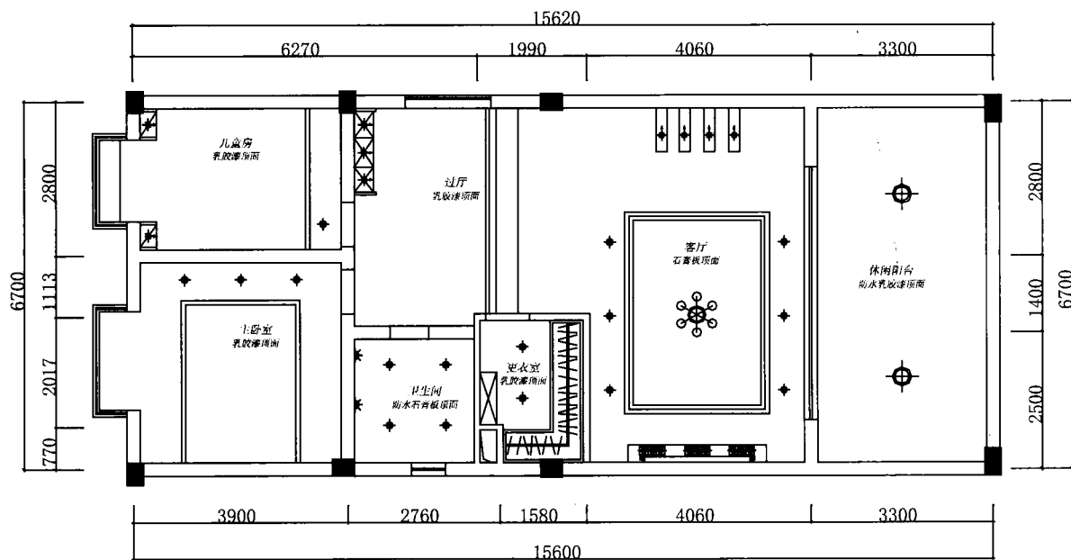
跃层设计
