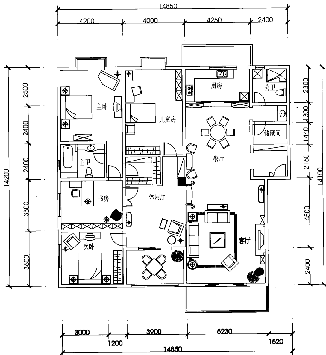
错层户型
