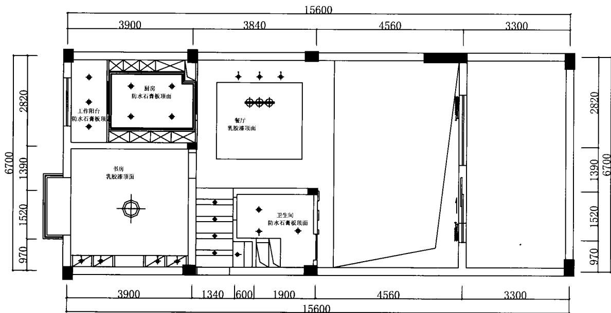
跃层设计
