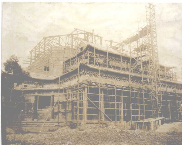
▶ 正在架设钢铁屋架的广州中山纪念堂建筑场景
