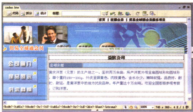
图 1-3 文档窗口
