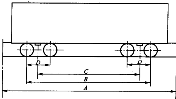
图 1-5 车辆轴距
