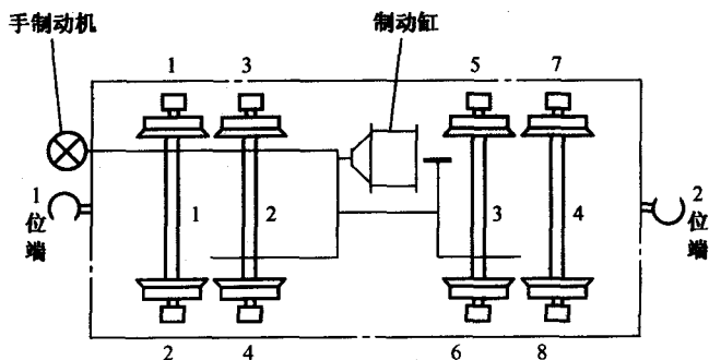
图 1-4 车辆方位
