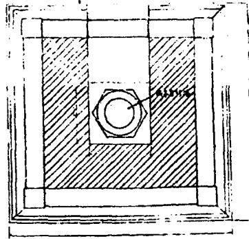
塔石平基
