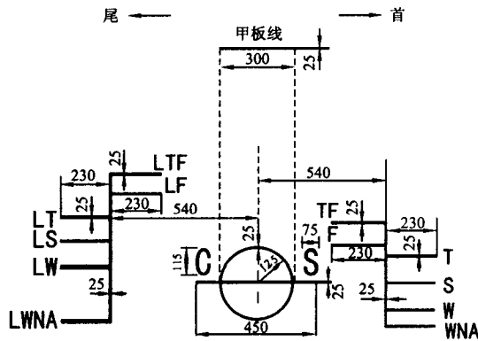
图 1-3 装载木材甲板货船舶的干舷及载重线标志 (单位: mm)
