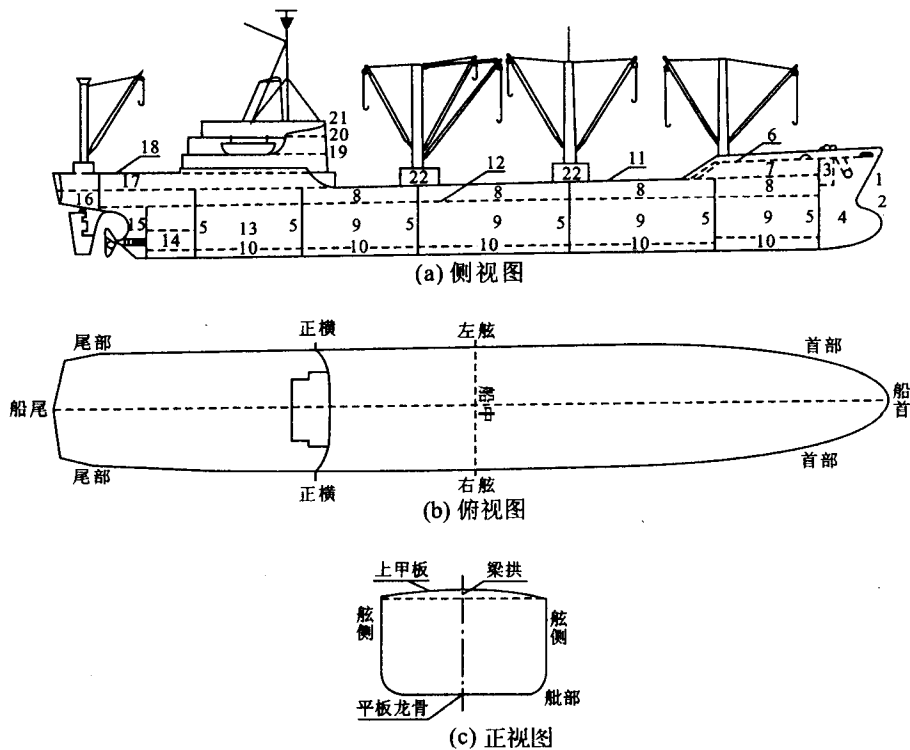
图 1-1 船舶各部位名称
