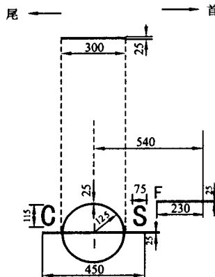
图 1-4 仅勘划淡水载重线标志的情况 (单位: mm)
