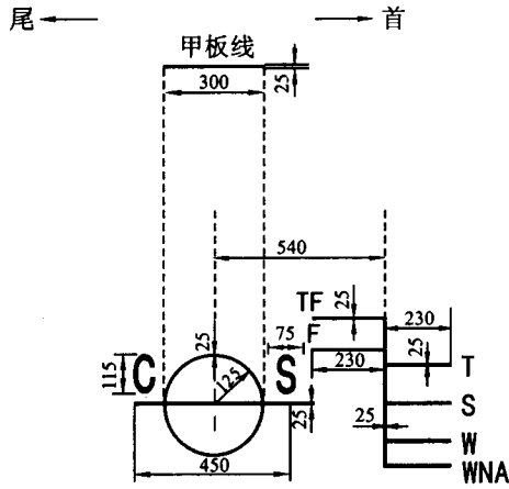
图 1-2 不装载木材甲板货船舶的干舷、载重线标志 (单位: mm)
