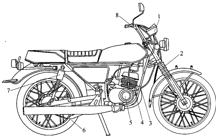
图 1-1 摩托车的组成
