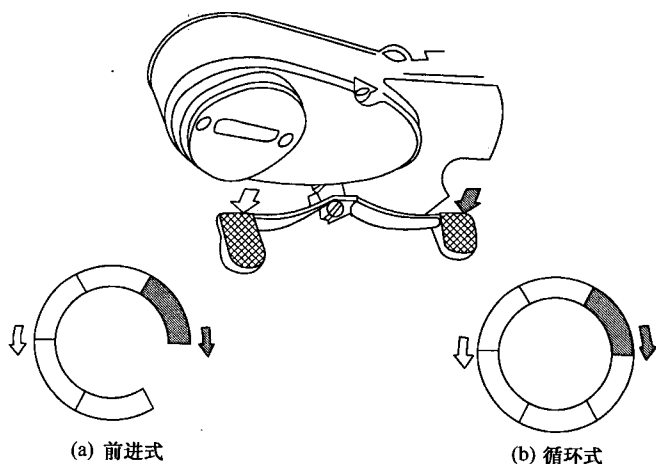
图 1-2 常见摩托车的排挡形式
