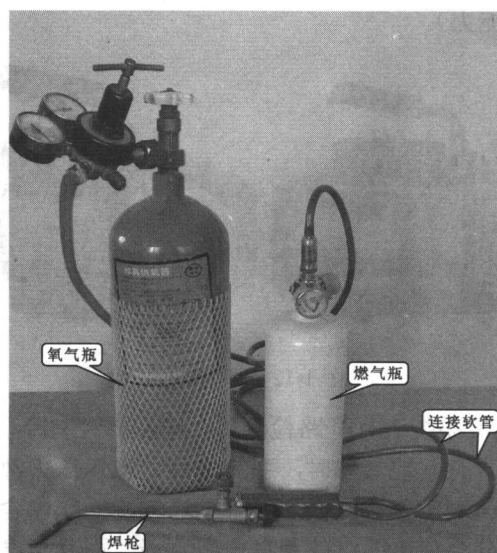
图 1-14 气焊设备
