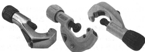
图 1-8 切管器
