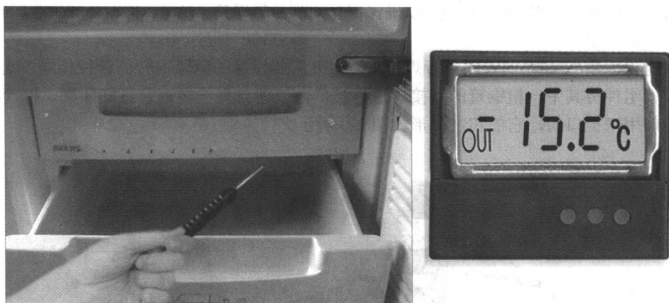
(a) 使用电子温度计检测电冰箱冷冻室的温度
