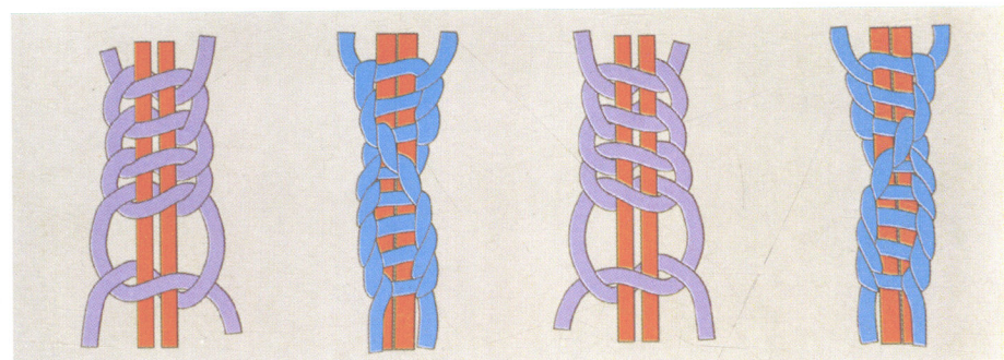
五、单平结(俗称死结)。
