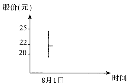
图 1-2 柱状图示意图
