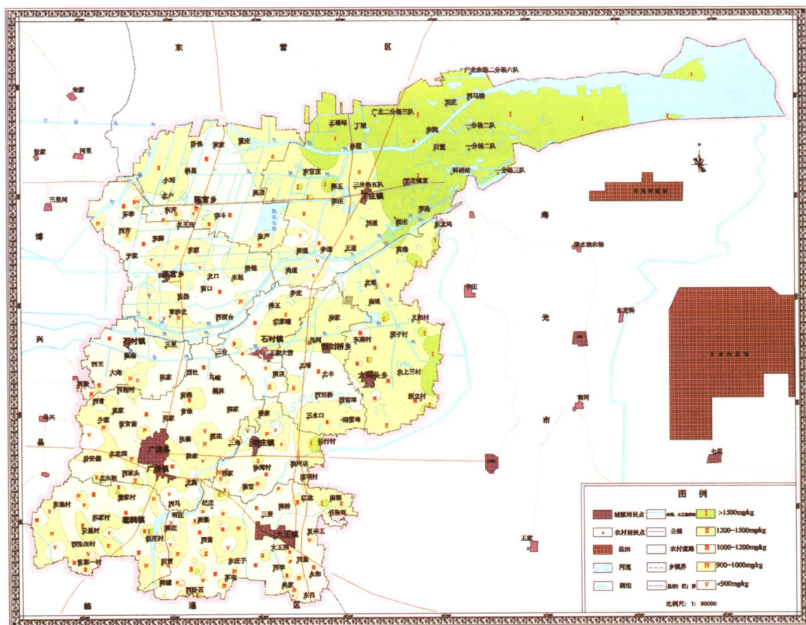
广饶县土壤缓效钾含量分布图
