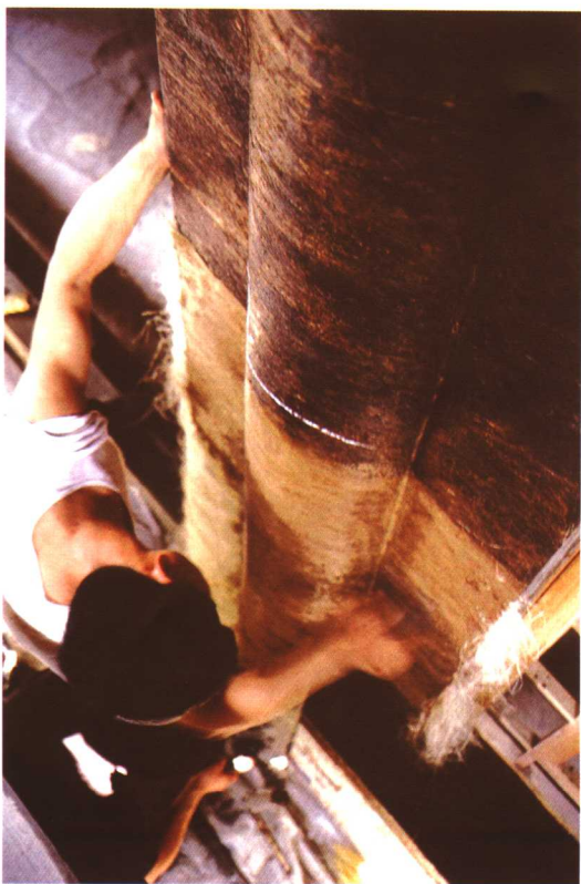
2 延春阁彩画做地仗工序披麻压麻
