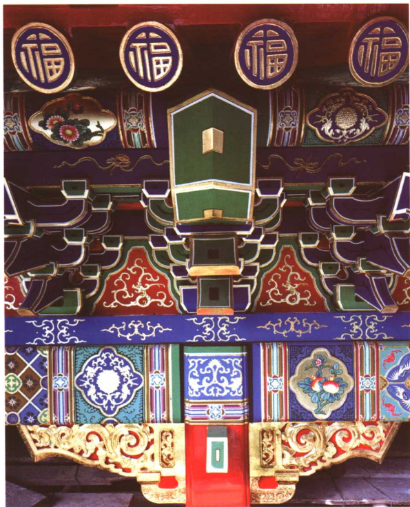
5 延春阁枋心式金线苏画
