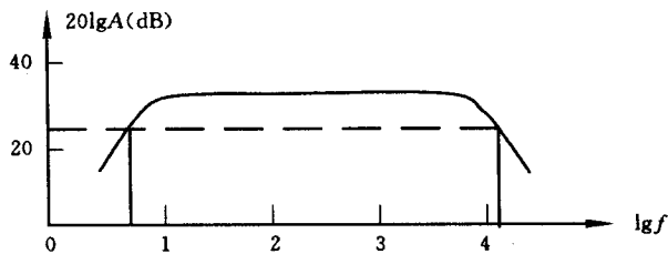
图 1-1-2 用双对数坐标绘制幅频特性
