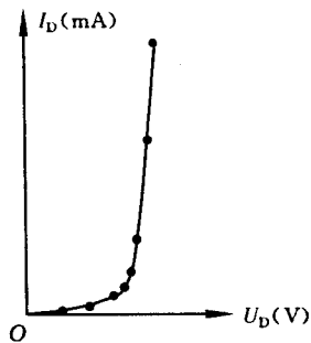
图 1-1-1 二极管特性曲线绘制
