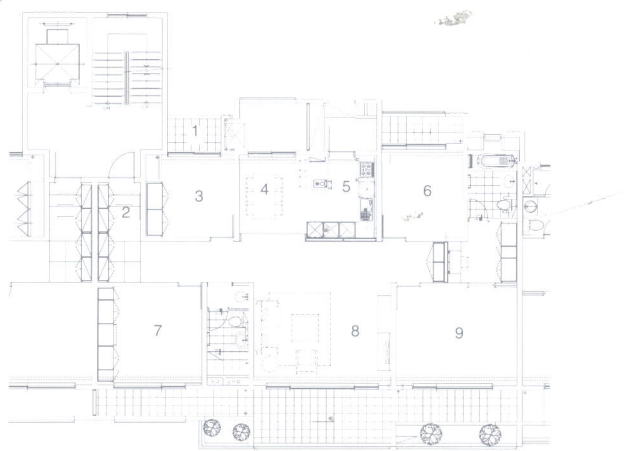
平面图
