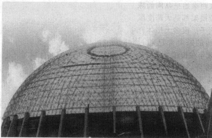
图 1-4 穹顶结构
