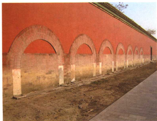
堆拨——现已被堵死，但券门仍在
