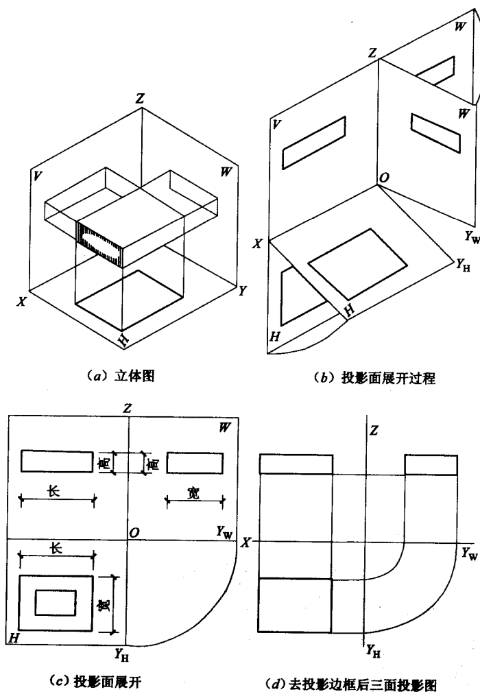
图 1-14 三面投影
