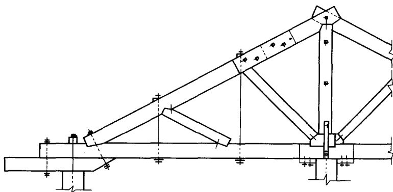
图 1-11 木屋架
