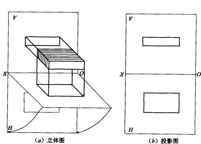
图 1-12 两面投影
