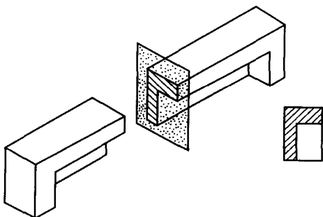
圖 1-20 剖面圖
