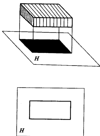
图 1-9 砖一面投影
