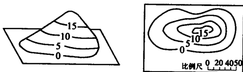
图 1-19 标高投影图 (m)
