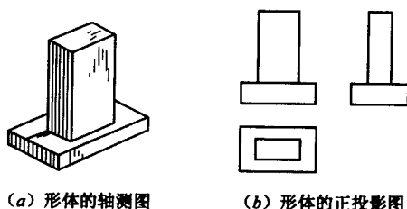
图 1-18 轴测图及正投影图
