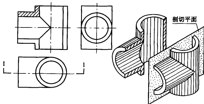
圖 1-22 全剖面圖
