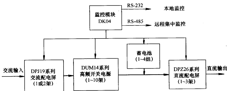
图 1-2 DUM14 高频开关电源系统构成框图
