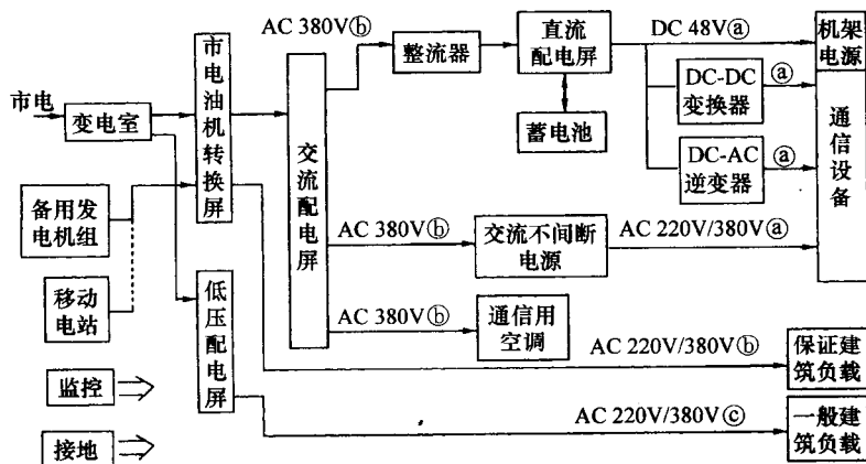
图 1-1 集中供电通信电源系统示意框图
