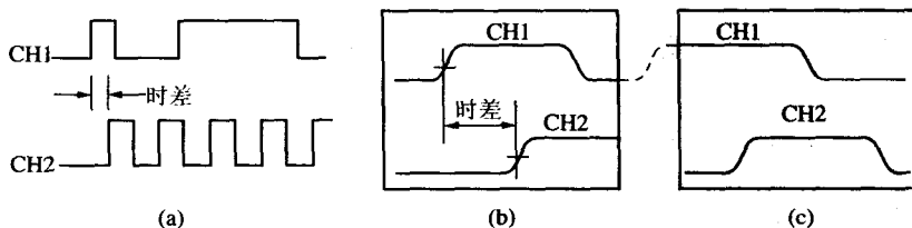
图 1.1.5 时间差测量波形图
