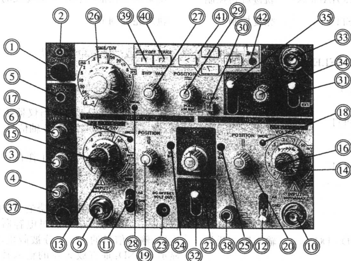
图 1.1.1 DF4325 型双踪示波器的前面板示意图
