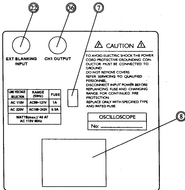
图 1.1.2 DF4325 型双踪示波器的后面板示意图
