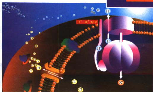
彩图6 质子泵的转运机制
