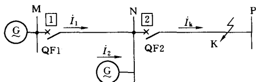
图 1-1 计算分支系数接线图
