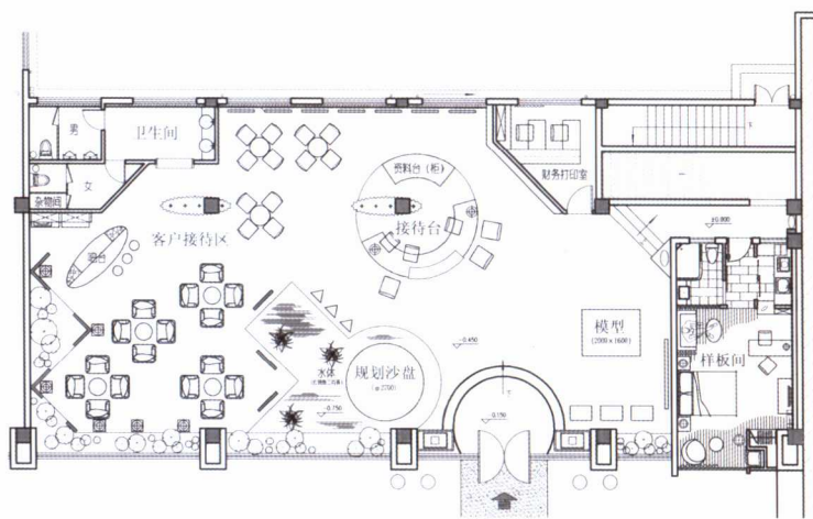
平面布置图
