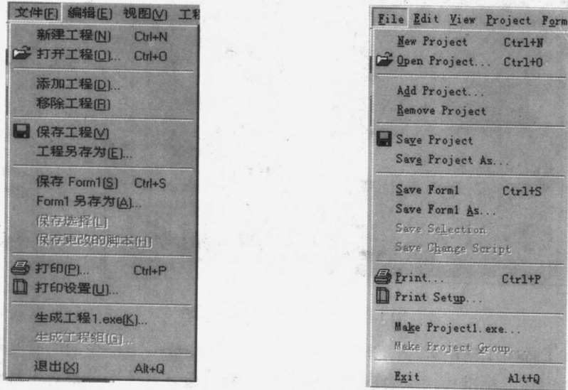
图 1.4 文件选单
