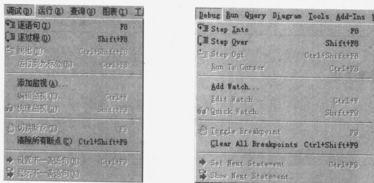
图 1.8 调试选单
