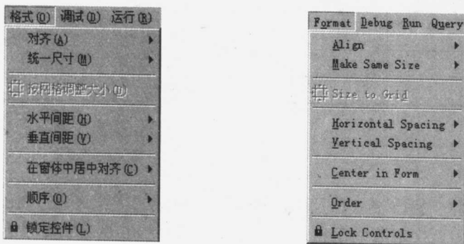
图 1.7 格式选单
