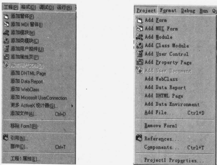
图 1.6 工程选单
